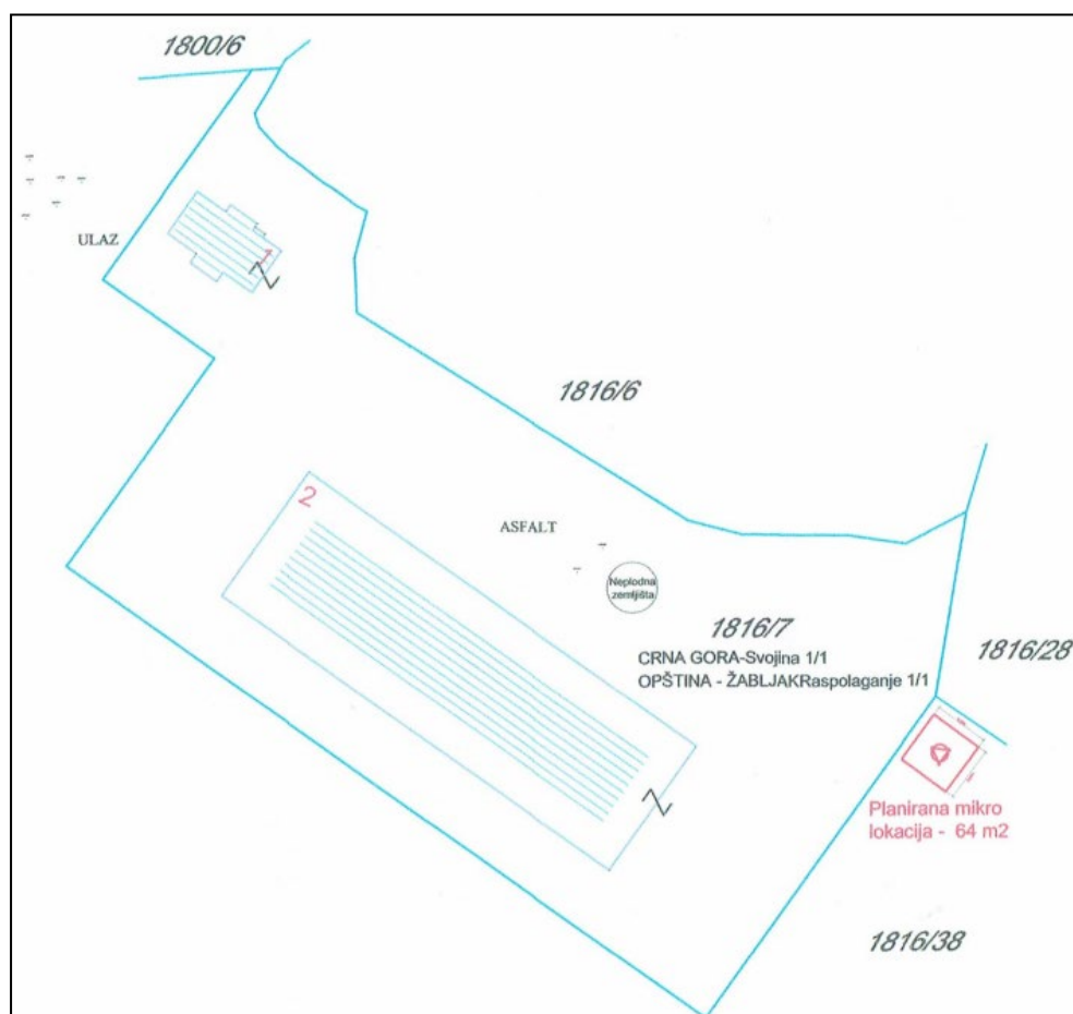
Slika 2.4. Skica prostora sa ucrtanim projektom
